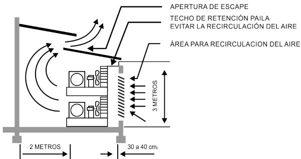
Abertura de escape = 2 veces a área de cara de 2 condensadores
