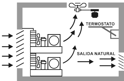
El extractor funciona cuando la temperatura interna alcanza el nivel para el cual el termostato está ajustado.
