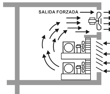
El extractor funciona con cualquier compresor ligado
